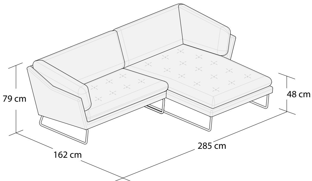
Narożnik lewy 2LM + OTMR
